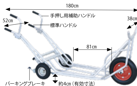
CU-1-3 アルミ製植木用一輪車 補助輪
