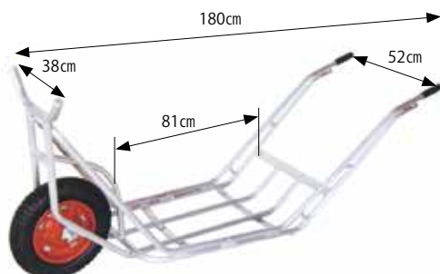
CU-1 アルミ製植木用一輪車
