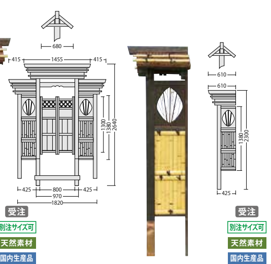
N-016 庭門 角柱Ⅱ型用片袖
