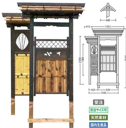
N-012 庭門 角柱片開Ⅱ型 片袖付
