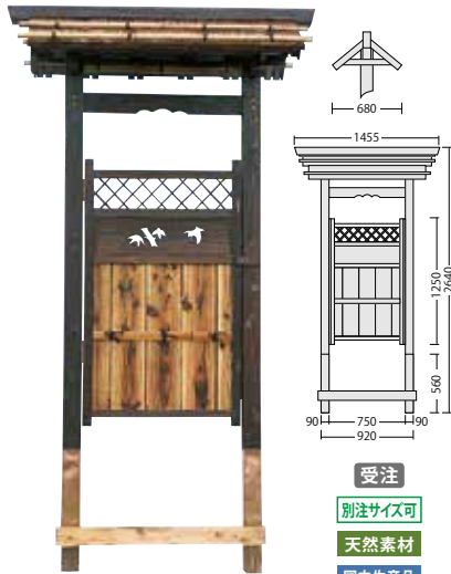
N-010 庭門 角柱片開Ⅱ型
