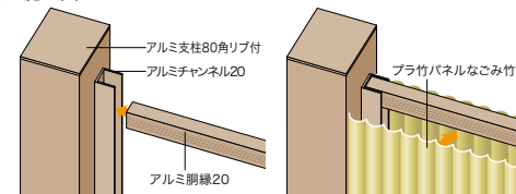
アルミ支柱80角リブ付ブラウン
