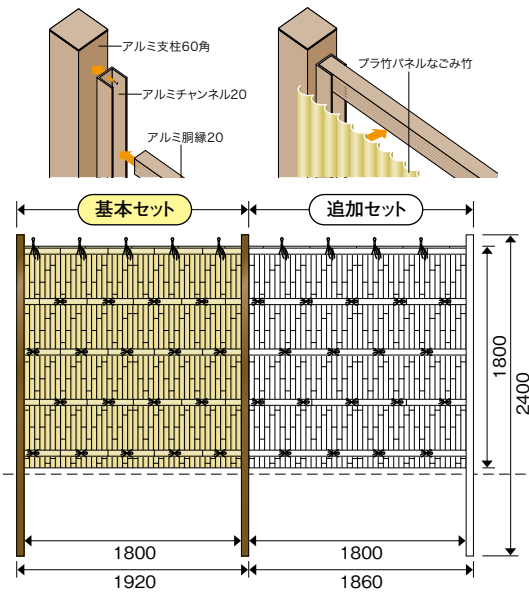
アルミ支柱60角ブラウン
