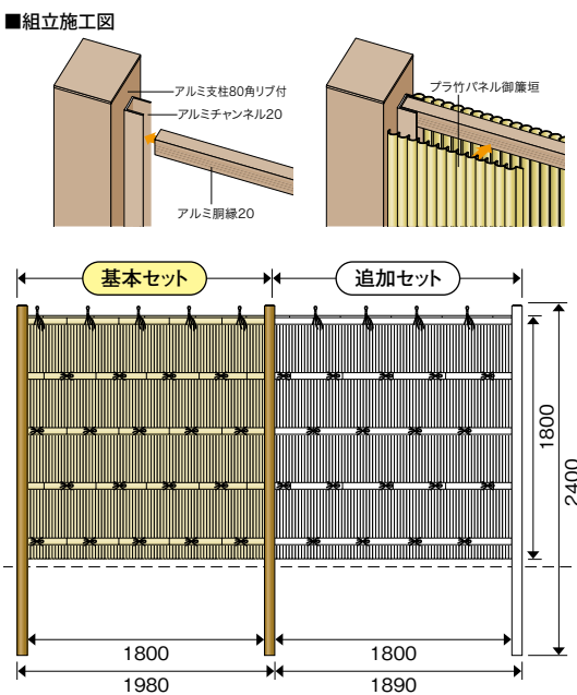
立御簾垣パネル イエロー 両面 アルミ支柱80角リブ付ブラウン使用 基本セット
