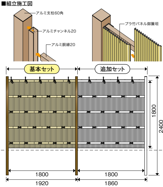
立御簾垣パネル イエロー 片面 アルミ支柱60角ブラウン使用 基本セット
