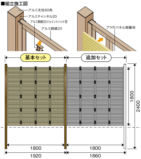
御簾垣パネル イエロー 片面 アルミ支柱60角ブラウン使用 基本セット
