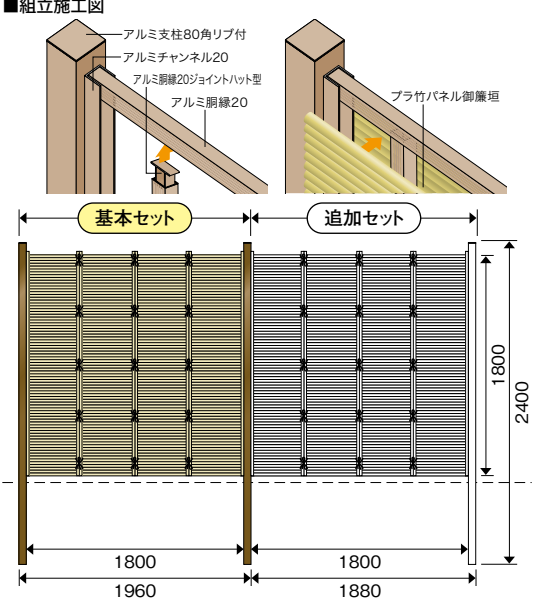
御簾垣パネル イエロー 両面 アルミ支柱80角リブ付ブラウン使用 基本セット
